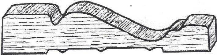
HC-313 * 11/16" x 3 1/2"
